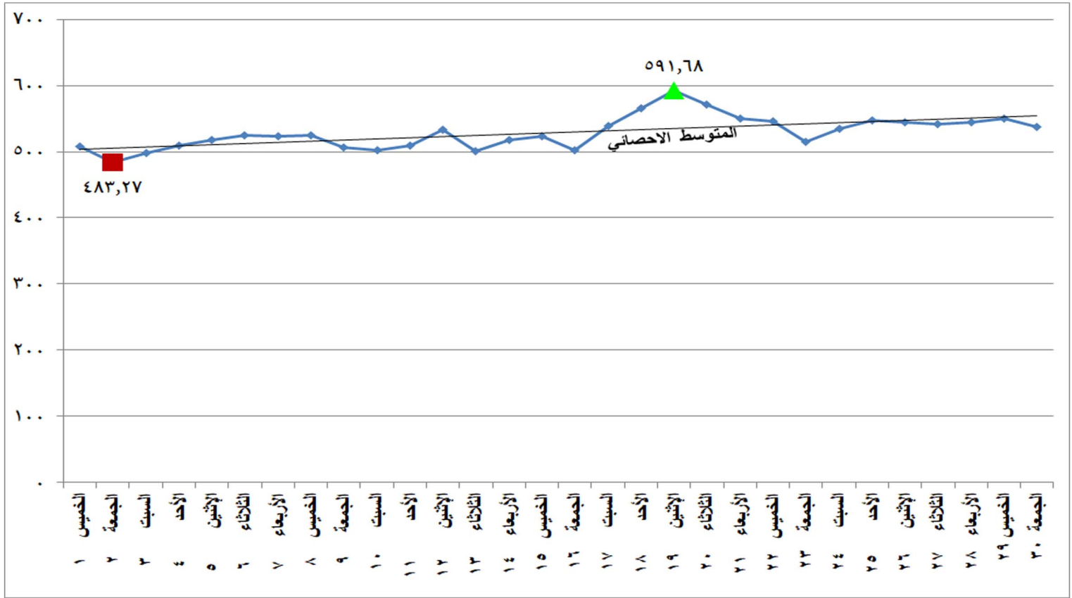
شكل (١٥) إجمالي الطاقة الكهربائية المنتجة من كل المصادر الأولية خلال شهر ابريل ٢٠٢١
