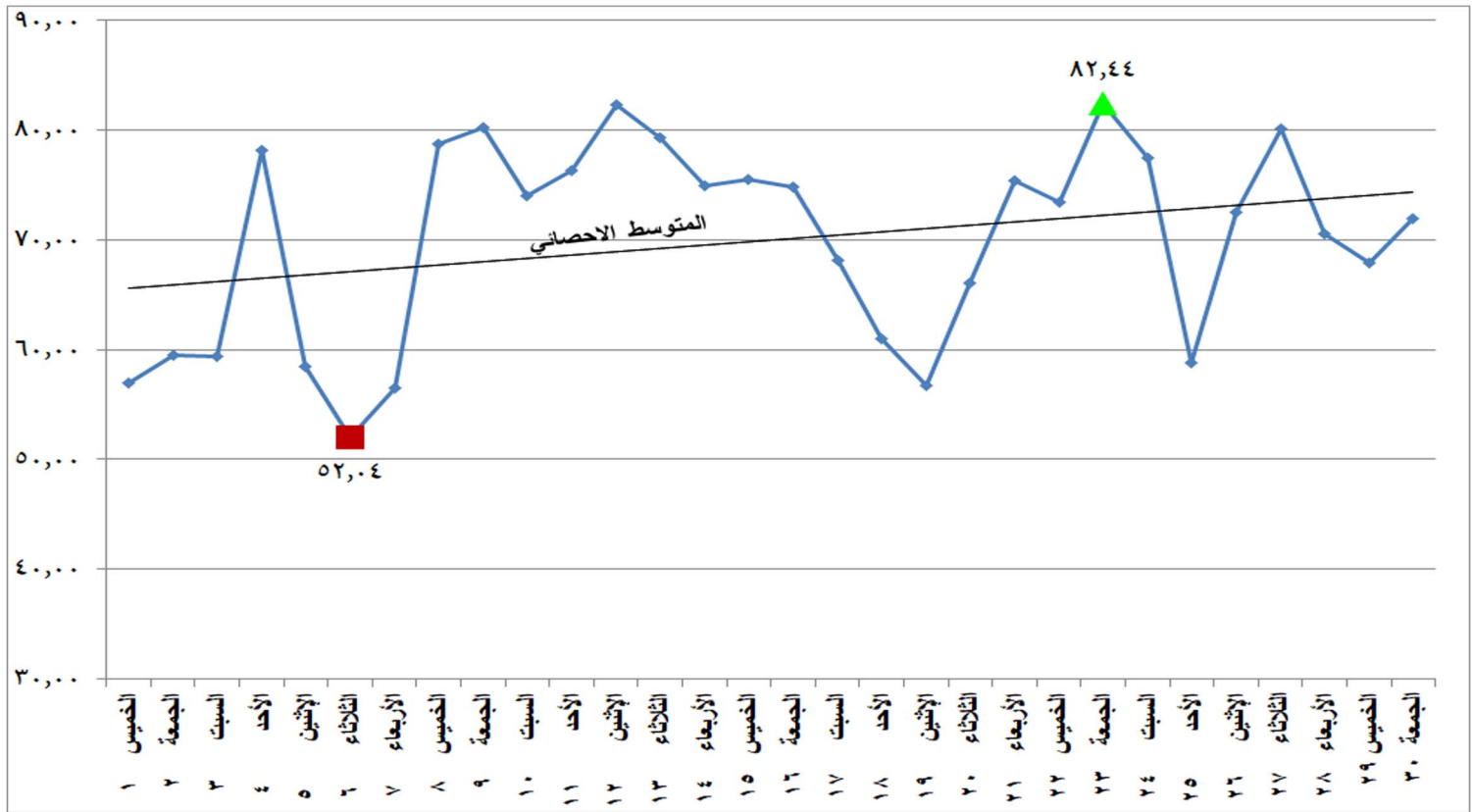
شكل (٢١) الطاقة الكهربائية المنتجة من المصادر غير الحرارية خلال شهر ابريل ٢٠٢١
