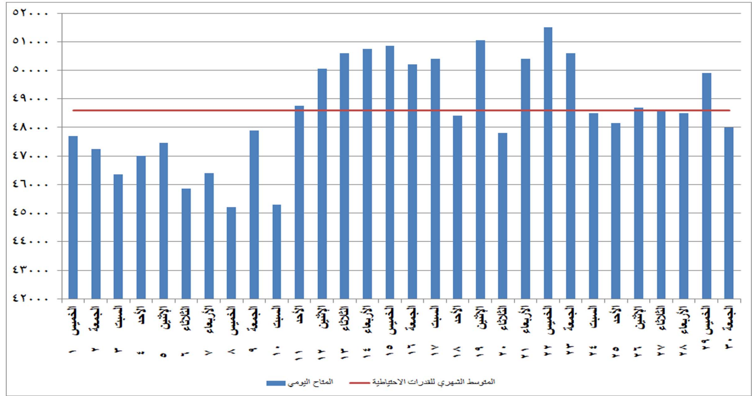
شكل (٢٧) القدرات المتاحة يوميا والمتوسط الشهري للقدرة الاحتياطية خلال شهر ابريل ٢٠٢١
