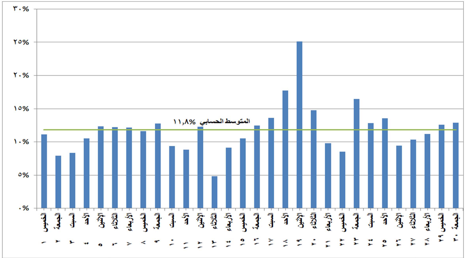
شكل (٩) النسب المئوية للتغير في الحمل الاقصى خلال شهر ابريل ٢٠٢١ مقارنة باليوم المماثل من العام الماضي
