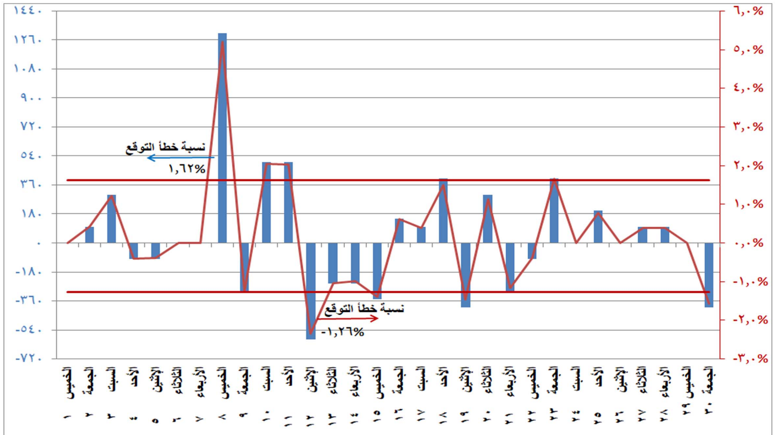
شكل (١٠) الفرق بين الحمل الأقصى المتوقع والمسجل فعليا ونسبة الفرق الى الحمل المسجل فعليا خلال شهر ابريل ٢٠٢١
