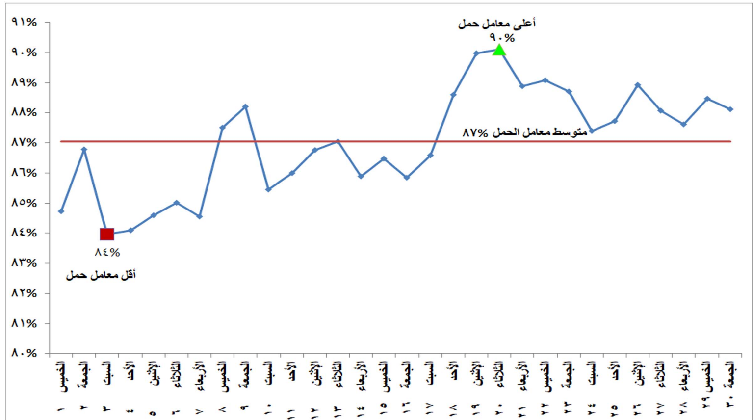
شكل (١٢) إجمالي معامل الحمل لوحدات الانتاج خلال شهر ابريل ٢٠٢١
