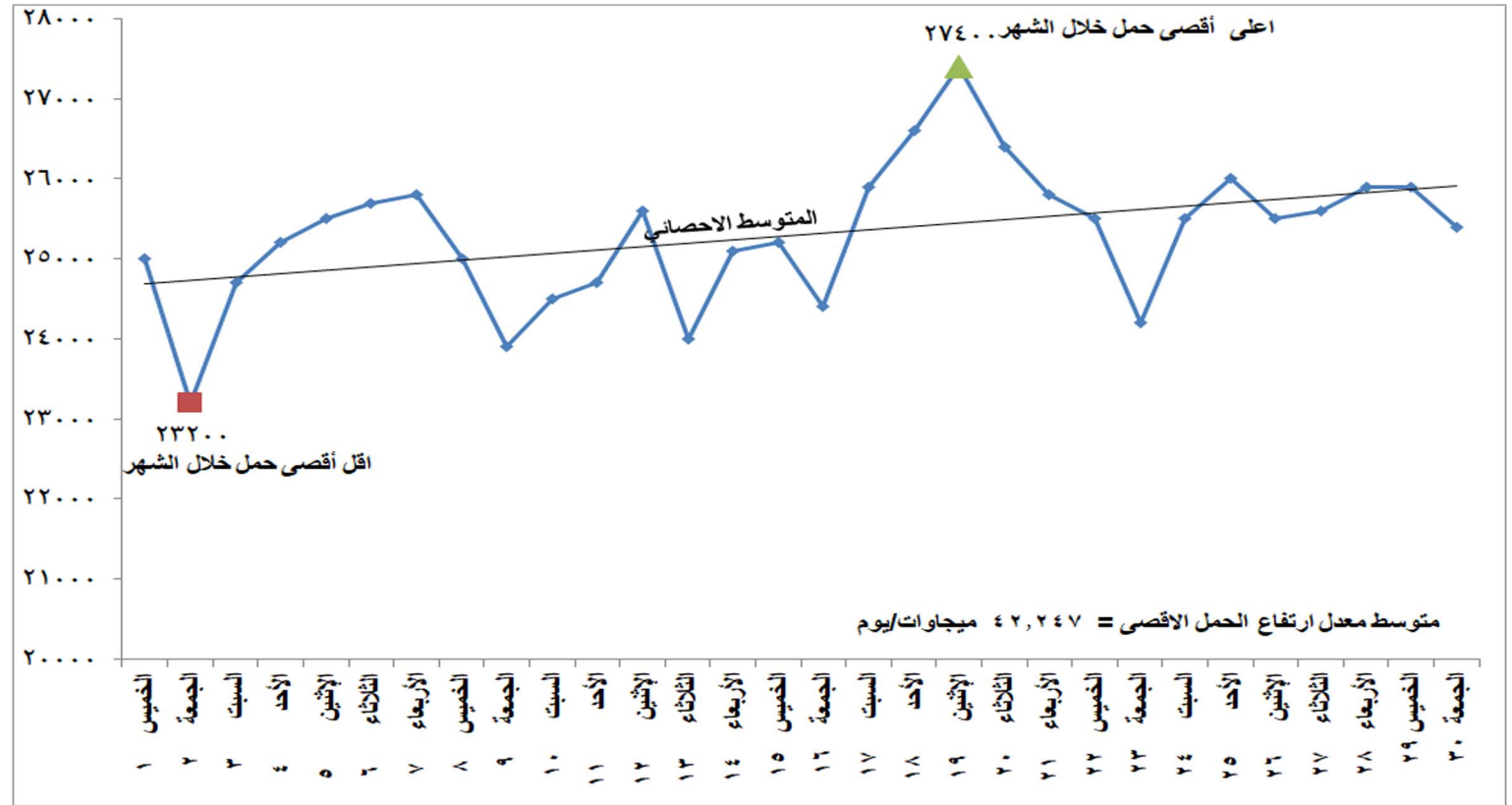
شكل (١) تطور الحمل الاقصى اليومي خلال شهر ابريل ٢٠٢١
