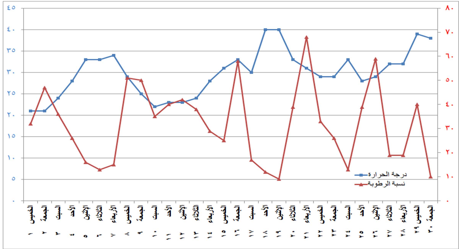
شكل (١١) التغيير في درجة الحرارة والرطوبة النسبية خلال شهر ابريل ٢٠٢١
