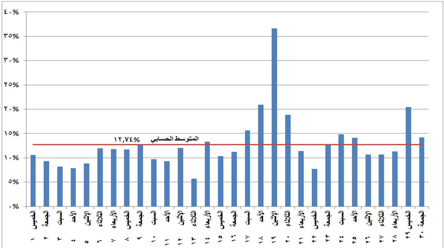
شكل (١٦) نسب التغير في الطاقة الكهربائية المنتجة خلال شهر ابريل ٢٠٢١ مقارنة بالشهر المماثل من العام السابق
