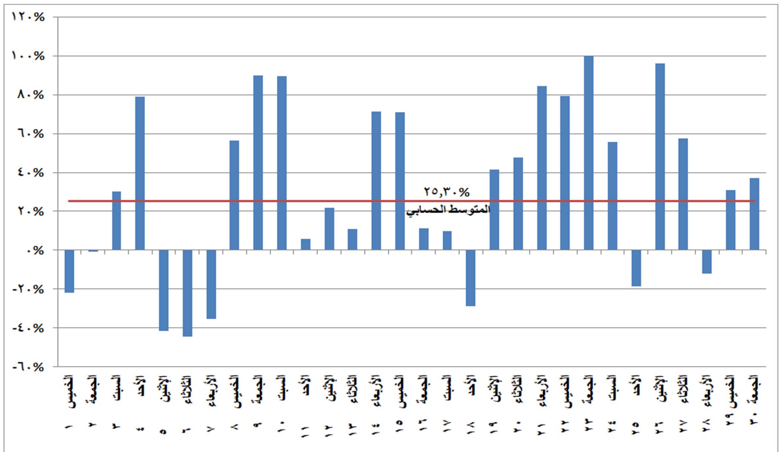
شكل (٢٦) نسب التغير في استخدام الرياح والشمس في إنتاج الطاقة الكهربائية خلال شهر ابريل ٢٠٢١ مقارنة بالشهر المماثل من العام السابق
