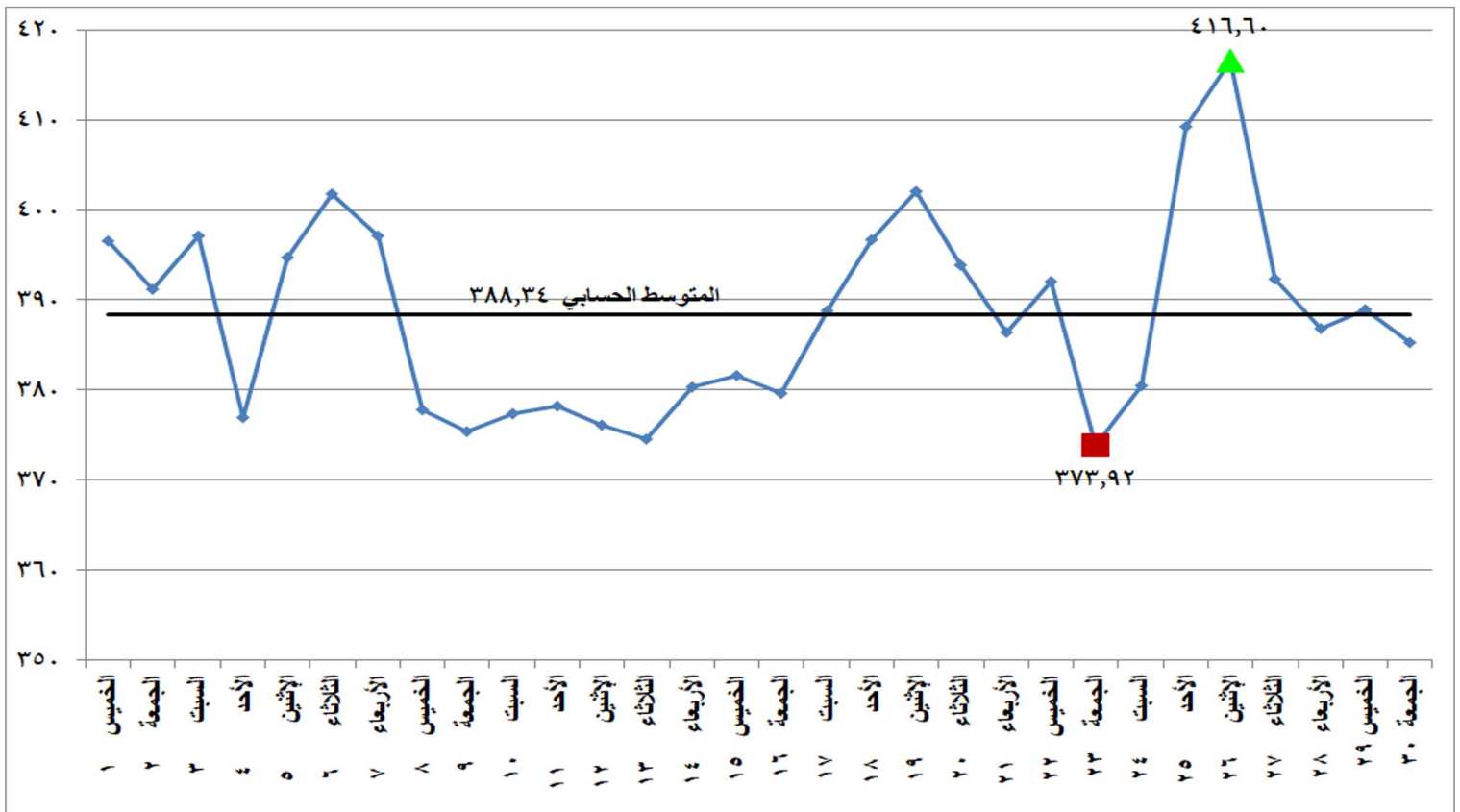
شكل (١٤) معامل انبعاثات غاز ثاني اكسيد الكربون المكافئ على مدى شهر ابريل ٢٠٢١
