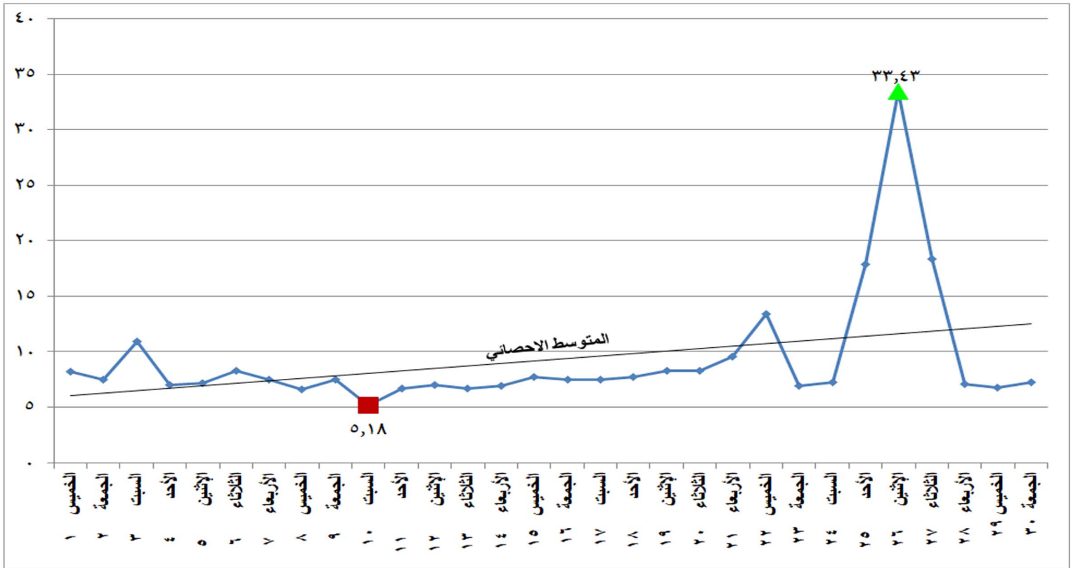
شكل (١٩) الطاقة الكهربائية المنتجة من المازوت خلال شهر ابريل ٢٠٢١
