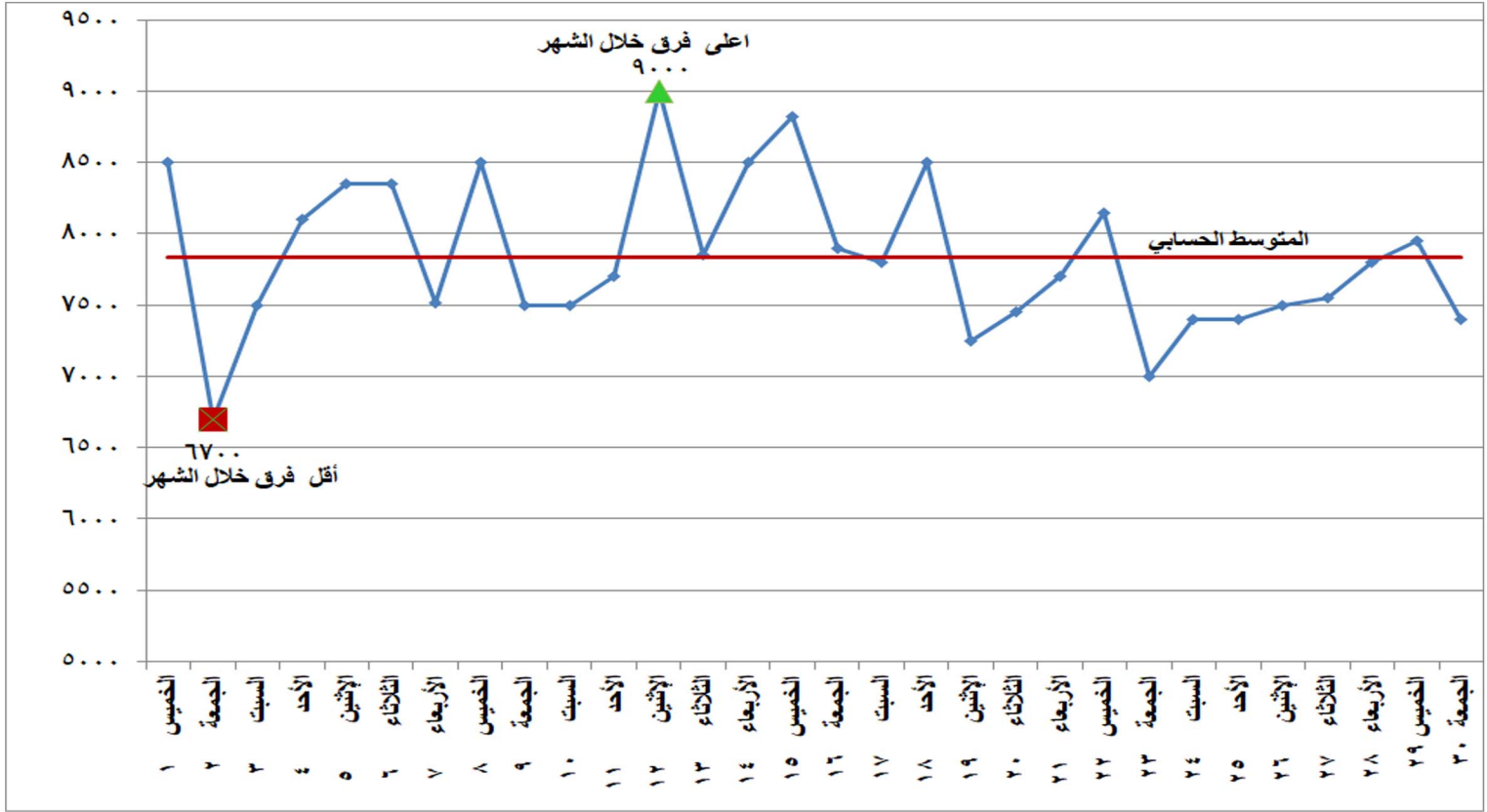
شكل (٣) الفرق بين أقصى وأدنى حمل خلال شهر ابريل ٢٠٢١
