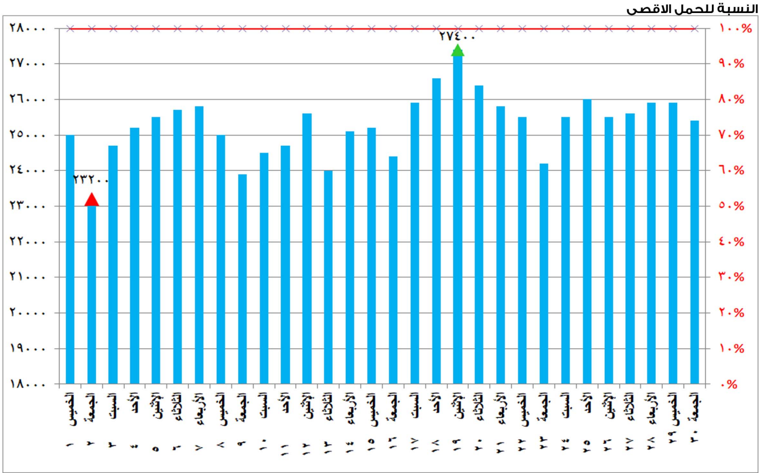
شكل (٥) قدرات الانتاج المتاحة ونسبتها للحمل الأقصى خلال شهر ابريل ٢٠٢١
